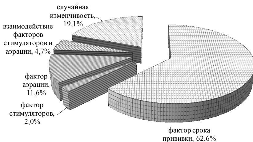
Рис. 2. Влияние факторов срока производства прививок, длительности аэрации при стратификации «на воде» и стимуляторов роста на выход черенков винограда с зачаточными корнями
