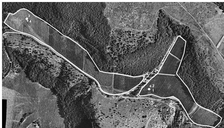
Рис. 1. Расположение экспериментальных площадок для оценки хлороза на винограднике UPPA: 1 и 3 – точки с развитием хлороза, 2 и 4 – контрольные точки без хлороза
