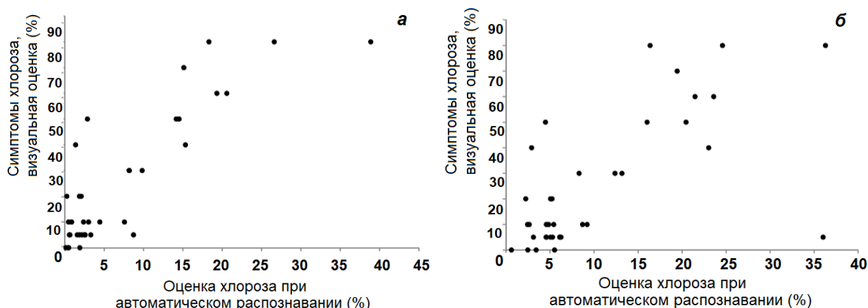
Рис. 5. Соотношение результатов визуальной и автоматической оценки хлороза при использовании двух алгоритмов распознавания фотоизображений (объем выборки 37): а – расчёт по алгоритму цветового пространства L^*A^*B ; б – расчёт по алгоритму цветового пространства H^*S^*V .
